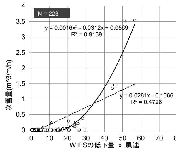
図2 画像評価値の低下量と風速の積と吹雪量の比較（春日テレメータ）
